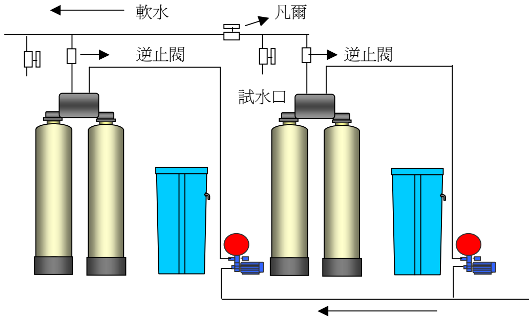
兩台並聯配置圖
